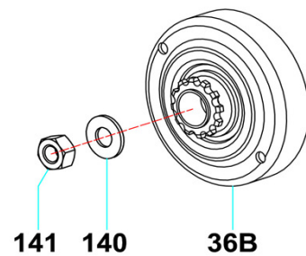
CAMPANA FRIZIONE Z12 Z12 CLUTCH DRUM
