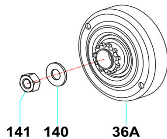
CAMPANA FRIZIONE Z11 Z11 CLUTCH DRUM
